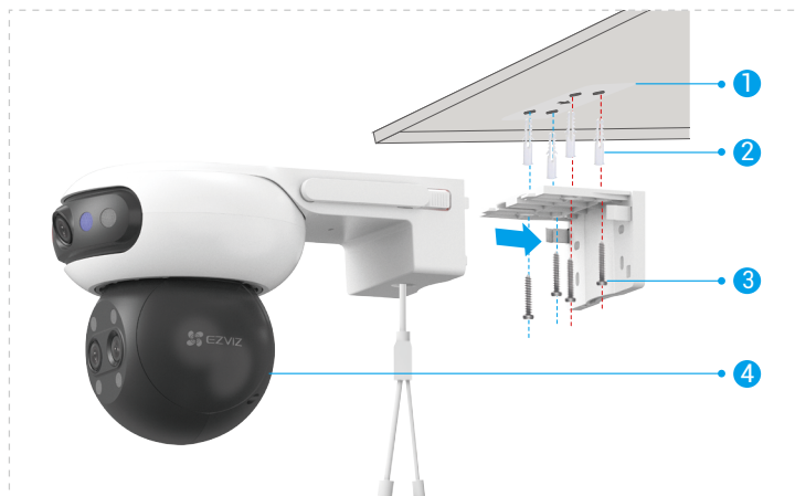
Abb. 1 Deckenmontage
